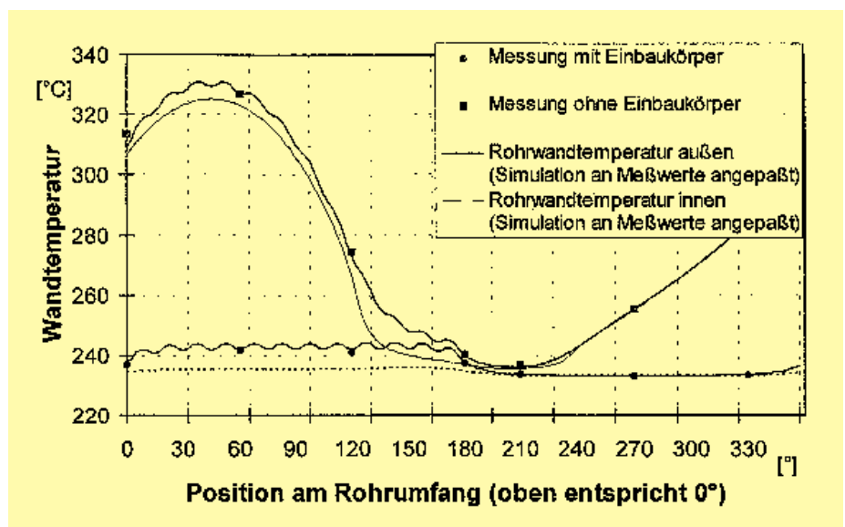
Abbildung 10: Rohrwandtemperaturverteilung für einen Versuchspunkt mit und ohne Einbaukörper ( \dot{m}_A = 57 \text{ kg/m}^2\text{s} , p = 30 \text{ bar} , \dot{q} = 56 \text{ kW/m}^2 seitlich)
