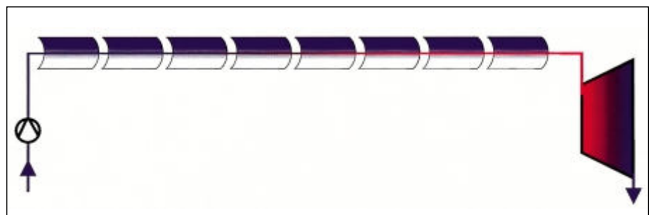
Abbildung 4: Direktverdampfung: Durchlaufkonzept
