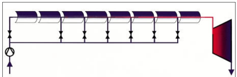
Abbildung 5: Direktverdampfung: Einspritzkonzept
