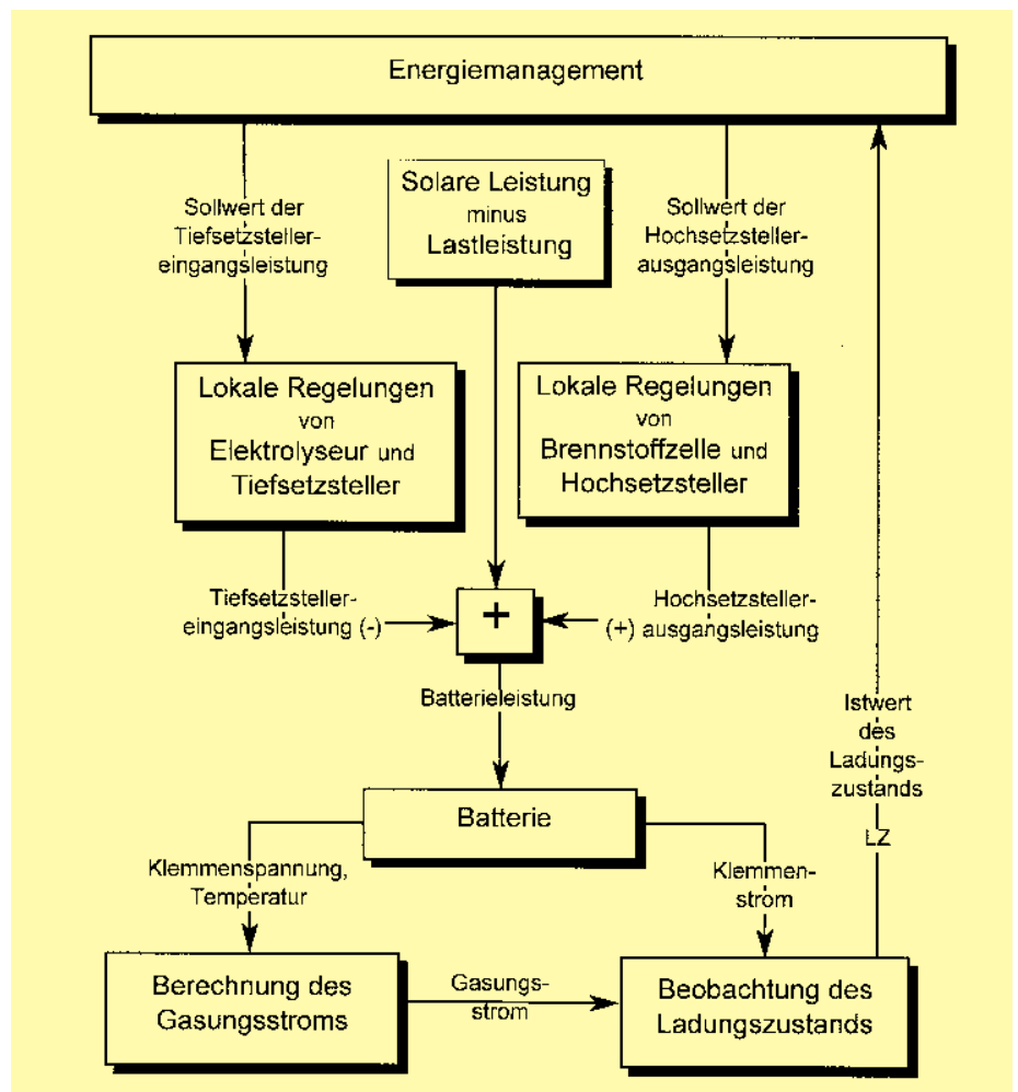
Abbildung 13: PHOEBUS-Regelkreis für den Ladungszustand. Nichtlineare Regler im Energiemanagement, Gleichstromsteller als ladungssteuernde Stellglieder, solare Leistung und Lastleistung als Störgrößen, implementiertes Modell zur Gasungsstromberechnung und numerische Integration des wahren Ladungsstromes.
