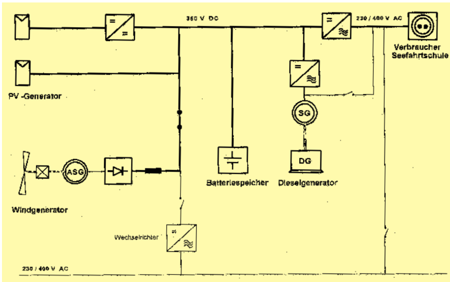
Abbildung 5: Prinzipieller Aufbau der Energieversorgung auf Terschelling. Die Hybridanlage auf Terschelling beinhaltet PV-Generatoren, einen Windgenerator, eine Batterie und ein Dieselaggregat zur Versorgung einer Seefahrt-Schule.
