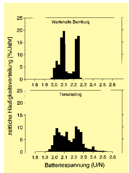
Abbildung 8: Häufigkeitsverteilung der Spannungen eines Jahres für die Anlagen Wartehalle Bernburg und Terschelling. Die Spannungsverteilung liefert Informationen über die Betriebsbedingungen der Speicher und das Einhalten von vorgegebenen Spannungsgrenzen.
