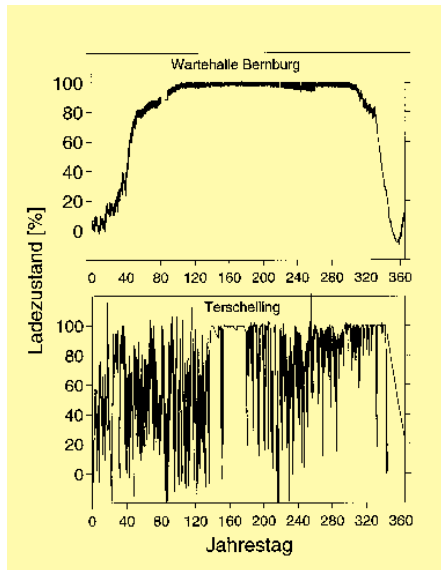
Abbildung 9: Ladezustandsverlauf über ein Jahr für die Anlagen Warte-halle Bernburg und Terschelling. Der Einsatz der Batterie der Warte-halle Bernburg als Wochen- und Monats-speicher gegenüber der von Terschelling als Tagesspeicher ist deutlich zu erkennen.
