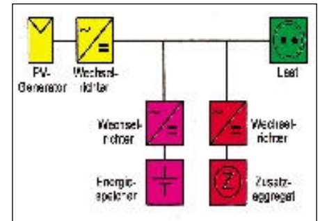
Abbildung 1: Blockschaltbild eines wechselstromgekoppelten Inselnetzes mit PV-Generator, Energiespeicher und Zusatzaggregat. Modulare Technologie beruht auf der Kopplung nach dem etablierten Wechselstromstandard.
