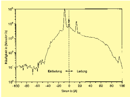
Abbildung 11: Die Häufigkeitsverteilung der Lade- und Entladeströme der Batterie für das Jahr 1995. Der mittlere Ladestrom von 20 A ist, bezogen auf die Nennkapazität von 1380 Ah, relativ gering. Der Entladungszeitraum unter 40 % betrug nur 300 h und mit einer Vollzyklenzahl von 44 ist eine hohe Lebensdauer zu erwarten.
