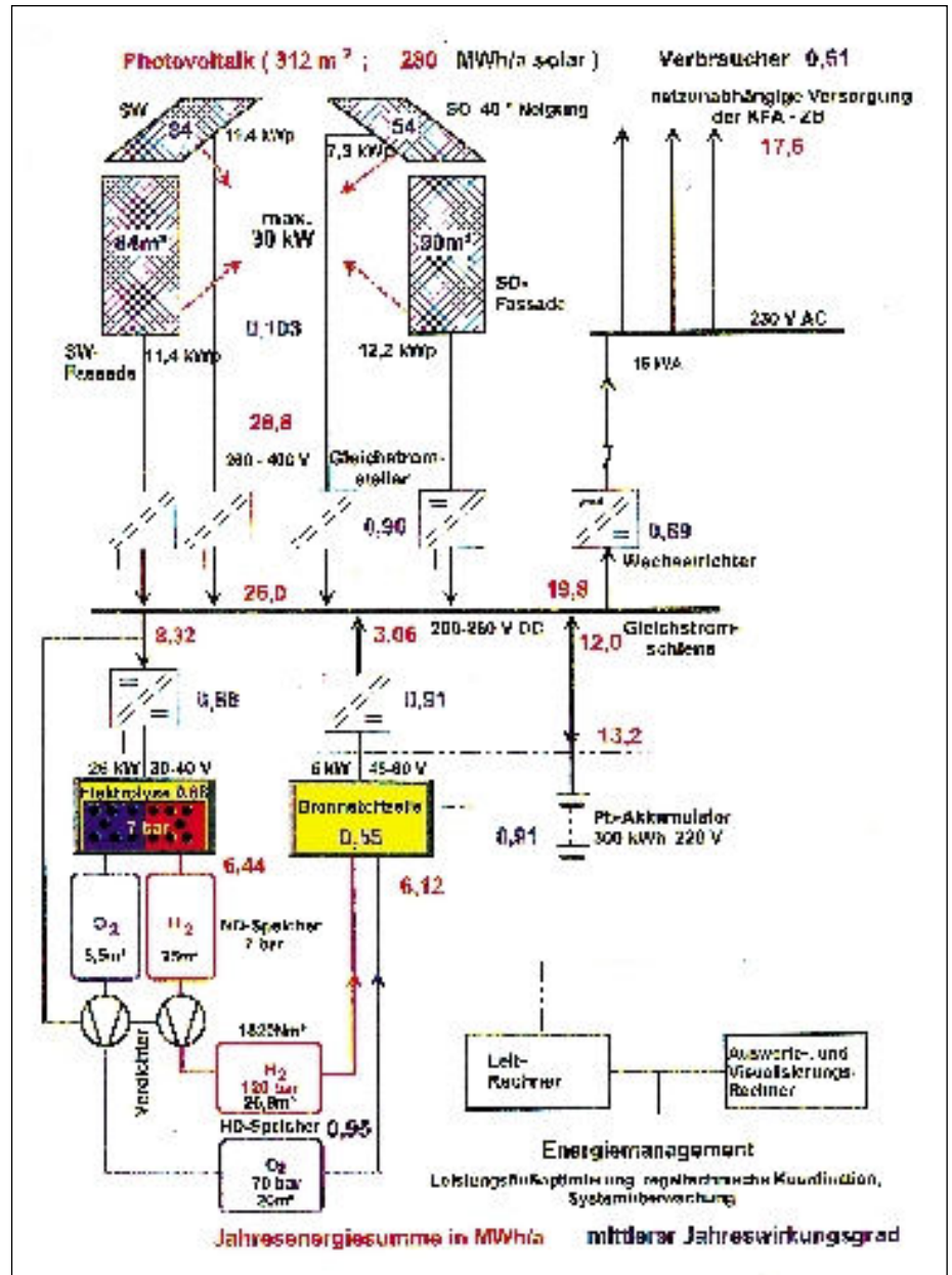
Abbildung 10: Die systemtechnische Konfiguration der PHOEBUS-Anlage mit den Jahresenergiesummen auf den einzelnen Pfaden und die mittleren Jahreswirkungsgrade der Energiewandlung in den einzelnen Komponenten.
