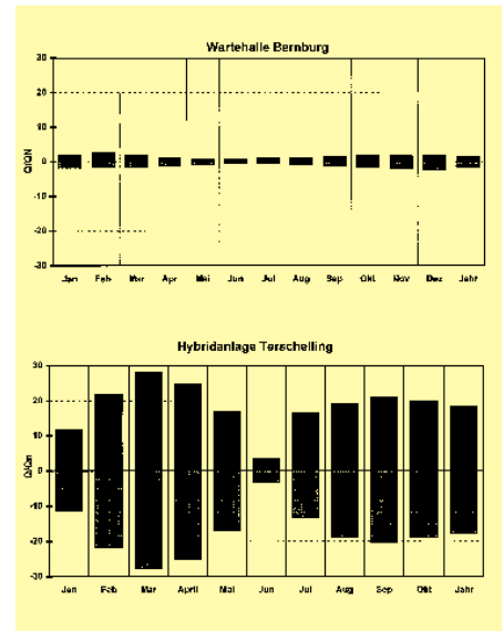
Abbildung 7: Monatlicher und mittlerer monatlicher Ladungsumsatz eines Jahres für Terschelling (360 V, 250 Ah) und Wartehalle Bernburg (12V, 56 Ah). Während die Batterie auf Terschelling im wesentlichen als Tagesspeicher eingesetzt wird, arbeitet die Batterie der Wartehalle Bernburg in den Wintermonaten als Wochen- und Monatspeicher.
