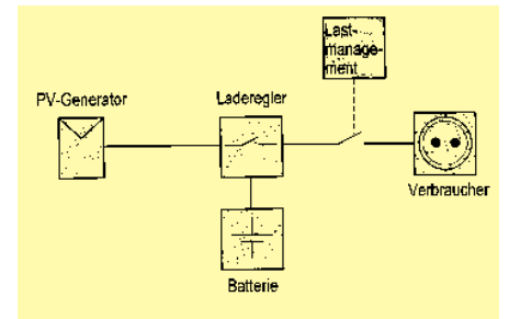
Abbildung 4: Prinzipieller Aufbau der Energieversorgung der Warte-halle Bernburg. Ein PV-Generator speist gleichspannungsseitig über einen Laderegler eine Batterie und eine Beleuchtung. Ein Lastmanagement optimiert den Betrieb.
