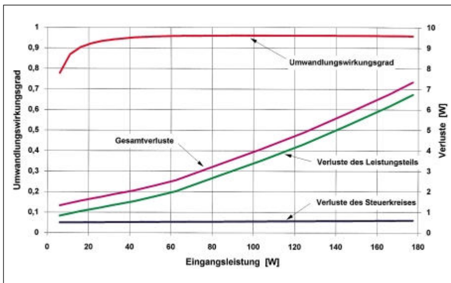
Abbildung 9: Gemessene Verluste und Umwandlungswirkungsgrad eines transformatorlosen Kleinwechselrichters zur Integration in die Anschlußdose von Dünnschicht-Solarmodulen. Durch konsequente Optimierung der freien Parameter lassen sich hohe Umwandlungswirkungsgrade von deutlich über 95 % in Verbindung mit guter Stromqualität auch mit Wechselrichtern geringer Leistung realisieren.
