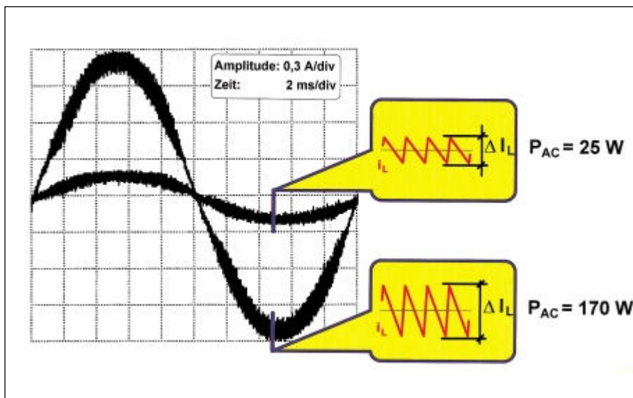
Abbildung 8: Gemessener Verlauf des eingespeisten Stroms bei Nennleistung und bei Teillast eines transformatorlosen Kleinwechselrichters für Dünnschichtmodule. Durch den Einsatz nichtlinearer Speicherdrosseln läßt sich eine Verringerung des Hochfrequenzanteils des eingespeisten Stroms im Teillastbereich erzielen. Zur Veranschaulichung wurden die Ströme bei einer stark verringerten Schaltfrequenz aufgenommen.
