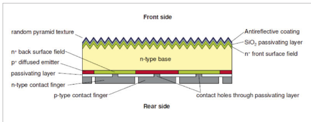
Abbildung 12 Rückseitenkontakt- solarzelle
