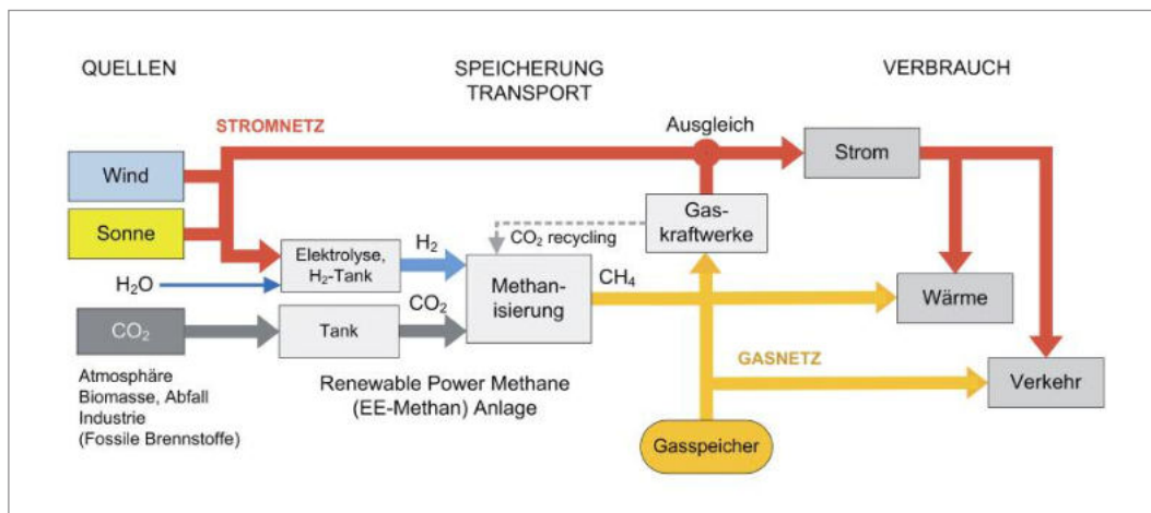
Abbildung 9 Erneuerbares Methan, Erzeugung und chemische Energie- speicherung
