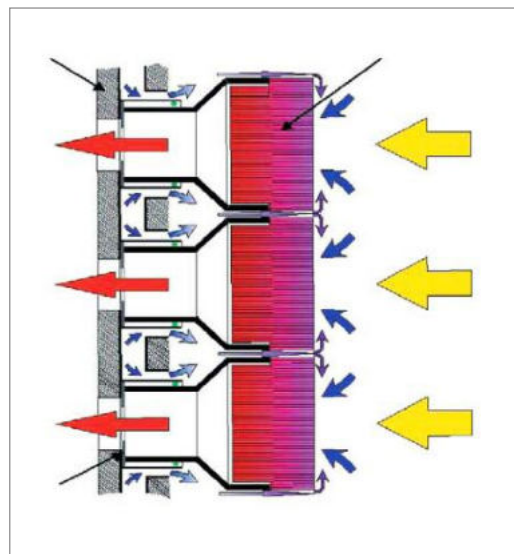
Abbildung 8 Volumetrische Solarreceiver, schematischer Aufbau des atmosphärischen Luftreceivers HITREC Quelle: DLR
