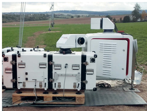
Abbildung 1 LiDAR-Scanner (links) und Messaufbau mit mehreren Multi-LiDAR- Systemen (rechts) für das Kassel- Experiment im euro- päischen Vorhaben „Neuer Europäischer Windatlas“ (NEWA) [Quelle: Fraunhofer IWES, Kassel]
