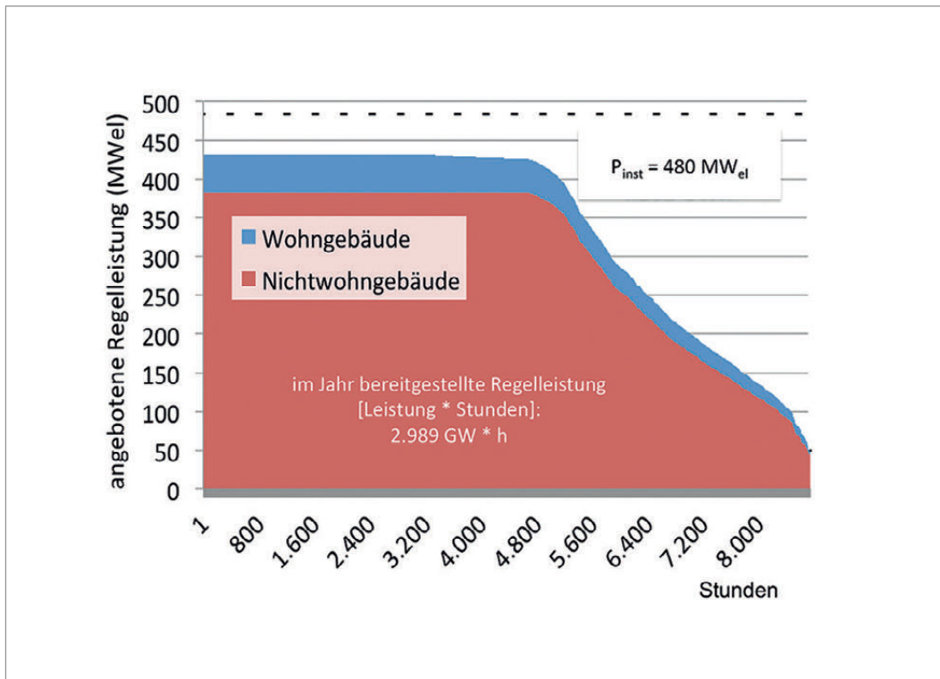
Abbildung 1 Modellierung: Jahresdauerlinie der potenziell bereit- gestellten Regelleistung für 2010
