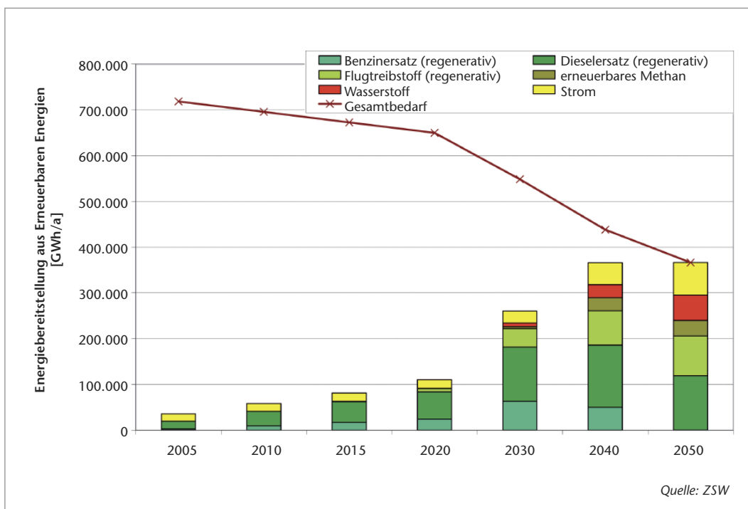
Abbildung 6c Entwicklung der Nutzenergiebereitstellung für Wärme aus erneuerbaren Energien und des Gesamtenergiebedarfs für Wärme in Deutschland bis 2050.
