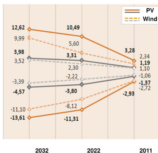
Max. Gradienten in DE durch PV* bzw. Wind**
