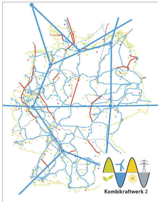
Abbildung 4 Szenarien zukünftiger Netzstrukturen mit Höchstspannungs- Gleichstrom- und Dreh- strom-Komponenten Quelle: Fraunhofer IWES et al, Pilotprojekt „Regeneratives Kombikraftwerk 2“, 2011/12
