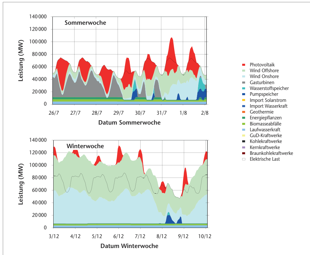
Abbildung 1 Stündliche Energie - bilanz in Deutschland in einer Sommerwoche (oben) und in einer Winterwoche (unten) im Jahr 2050 für ein Szenario mit 90 % jähr- lichem erneuerbarem Energieanteil an der Stromversorgung auf der Basis überwiegend variabler erneuerbarer Quellen.
