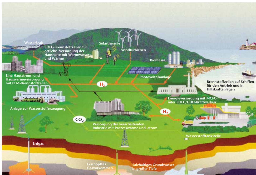
Abbildung 1 Darstellung einer „Wasserstoffwelt“ als Energiemix aus Erdgas und erneuerbaren Energien
