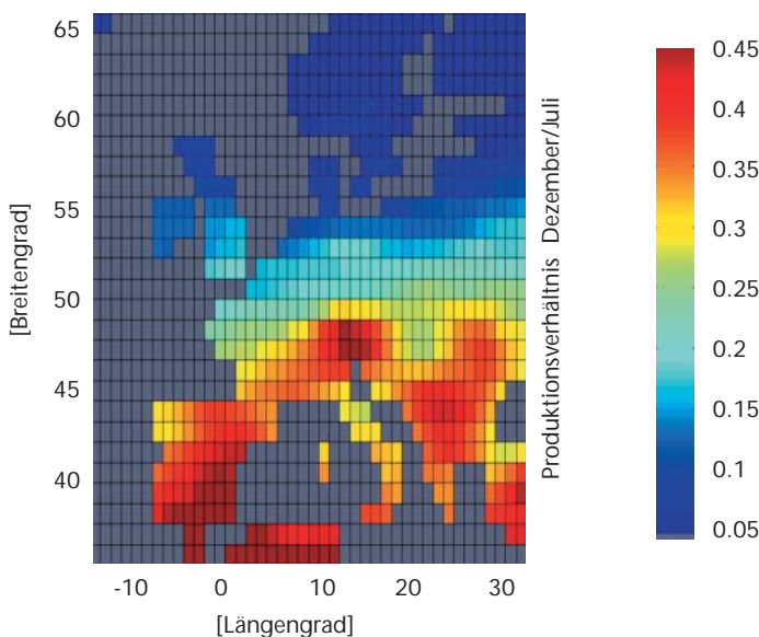
Abbildung 6 Saisonaler Vergleich der mittleren Stromproduktion aus Photovoltaik, Quotient aus Monatsmittelwerten der Dezember- und Julierzeugung 1983-1992; met. Daten: EZMW und NCEP.
