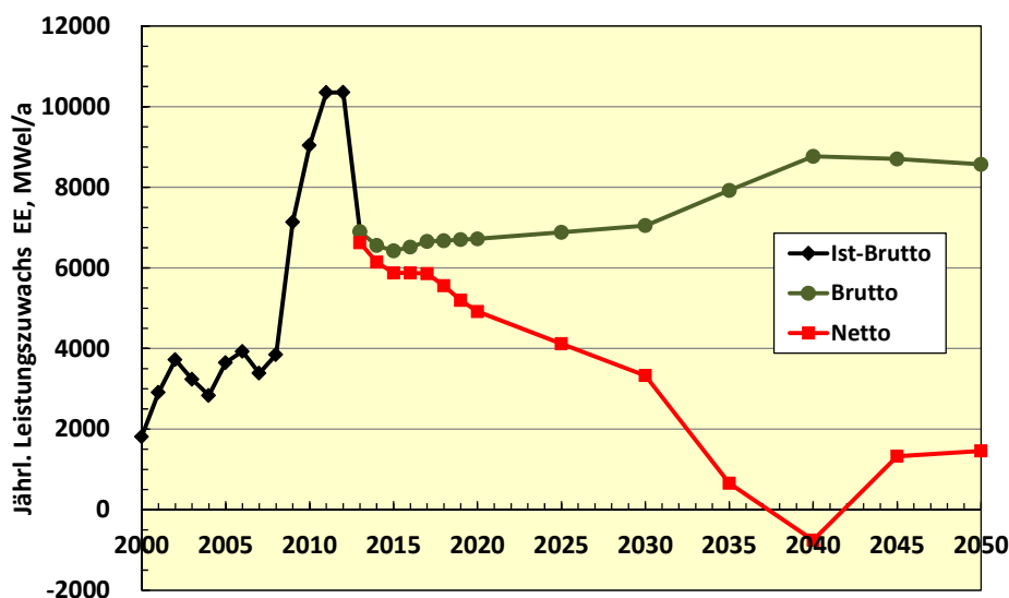
Abbildung 5: Brutto- und Nettozubau aller EE- Anlagen zur Stromerzeugung im Szenario GROKO-II
