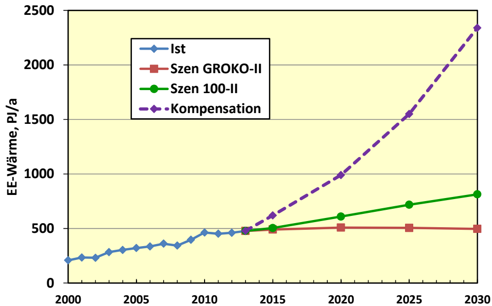
Abbildung 21: Wachstum des EE-Wärmebeitrags in den Szenarien GROKO-II und 100-II und erforderliche zusätzlicher Zubau (Kompensation), wenn die CO 2 -Minderungsziele bei unzulänglichem KWK- und EE-Stromwachstum (aber ausreichender Effizienz) erreicht werden sollten.
